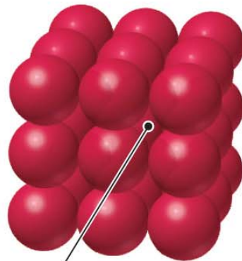
Simple cubic
