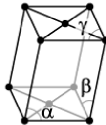
Monoclinique centré
